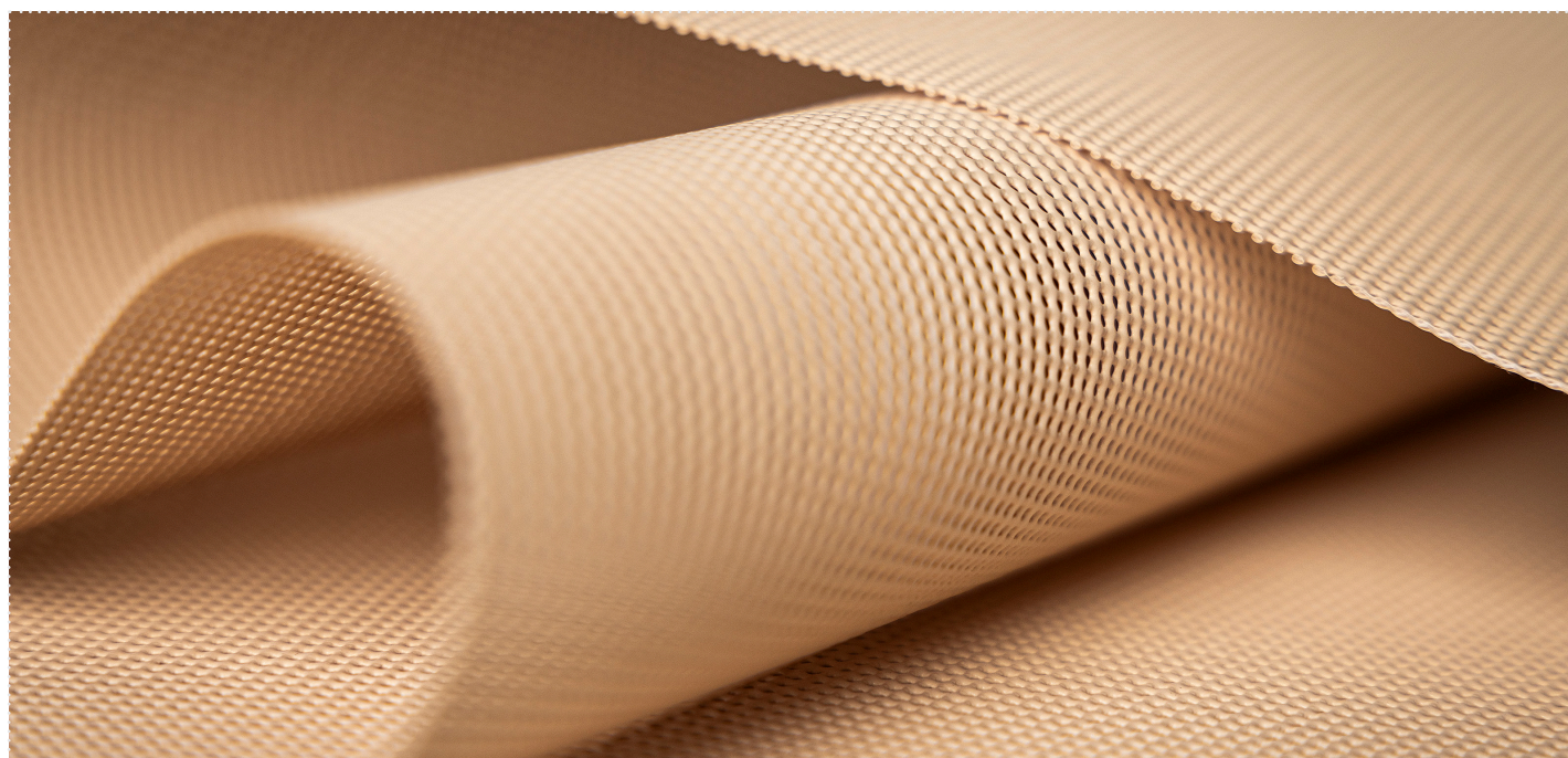
Structura 230 - 1815 (sandstone)
